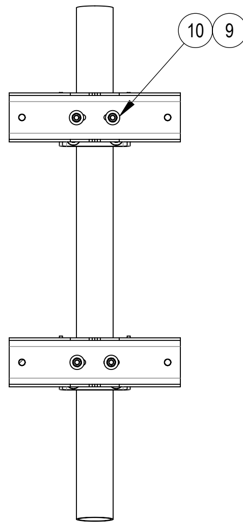
SECTION A-A
