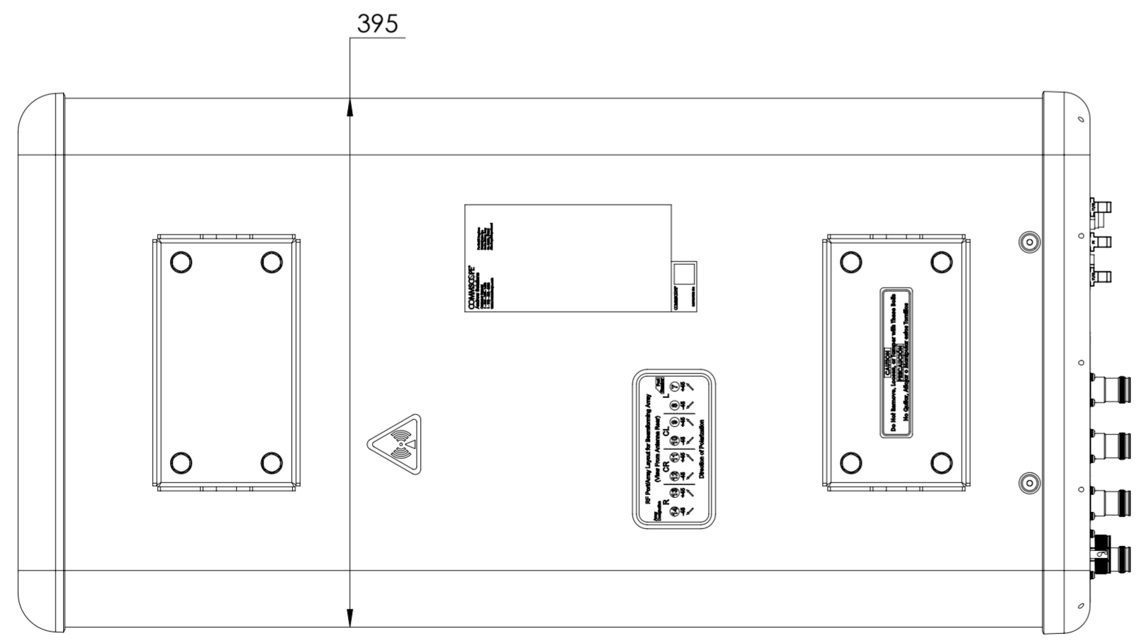
RVVS4-65S-R3
