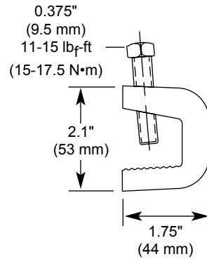
C Snap-in cable hanger Soporte colgante de cable de inserción inmediata Support de câble à fixation immédiate Schnappkabelhalter Abraçadeira para cabos Snap-In 咬接式电缆挂钩
